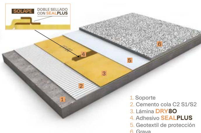
cubierta no transitable con grava
