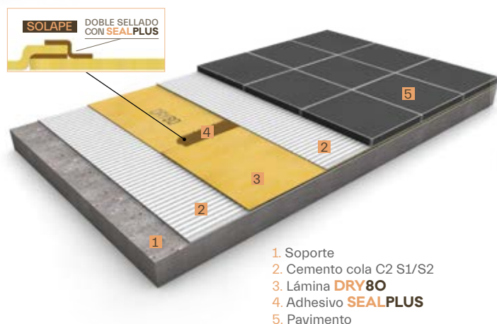
cubierta transitable con pavimento
