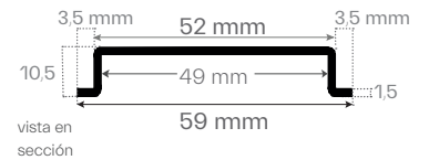
D/D_base canaleta
