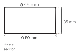
D/D_base canaleta
